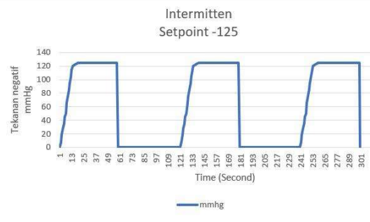
Gambar 4.13 Grafik mode intemitten setpoint -125
