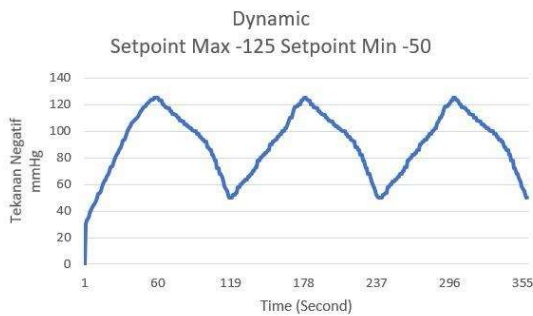
Gambar 4.17. Grafik mode dinamis setpoint -125
