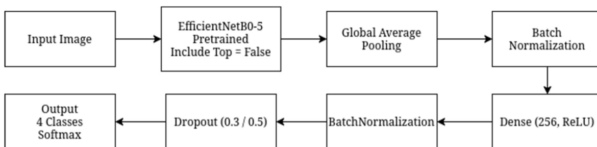
Gambar 4. Arsitektur Model
