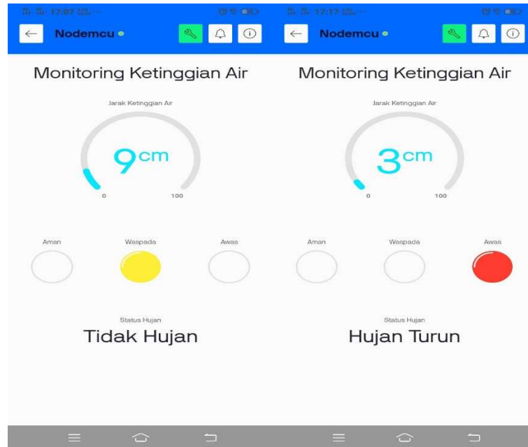
Gambar 5. Tampilan Aplikasi blynk saat pengujian rangkaian
